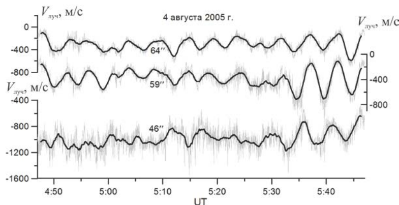
Рис. 1. Пример осциллограмм трех временных последовательностей значений лучевой скорости, измеренных в линии FeI 6569 Å
