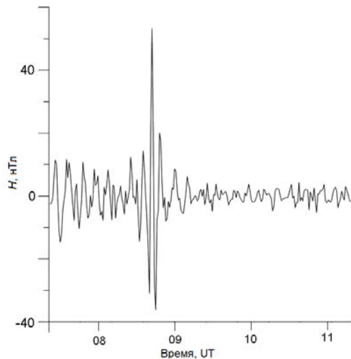
Рис. 2. УНЧ-колебания в диапазоне Pc5, зарегистрированные на обс. «Мирный» 04.01.1988 в весьма спокойных геомагнитных условиях: K_p = 1 [Зотов и др., 2013]
