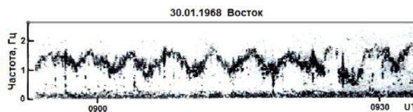
Рис. 1. Динамический спектр колебаний Pc1 с глубокой модуляцией несущей частоты [Guglielmi et al., 2015]
