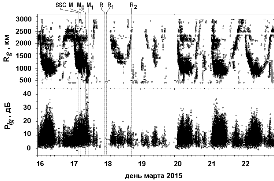
Рис. 4. Для 16–22 марта 2015 г. показаны вариации дальности R_g и мощности P_{lg} сигналов, рассеянных неоднородностями земли.
