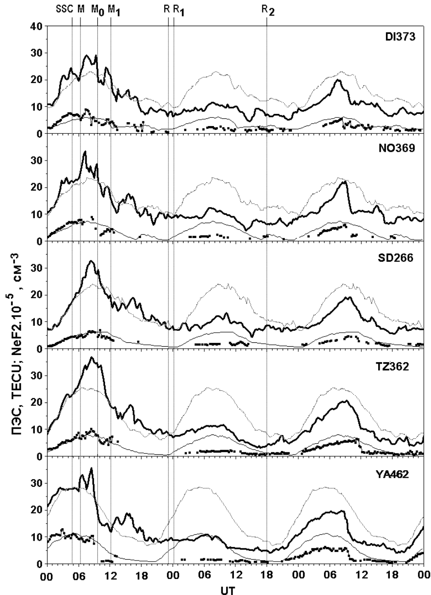
Рис. 6. Вариации ПЭС и электронной концентрации N_m F_2 в максимуме F2-слоя над пятью ионосферными станциями. Названия станций указаны на панелях. Текущие и фоновые значения ПЭС показаны, соответственно, толстой и точечной линиями; N_m F_2 — тонкой линией с квадратами и тонкой линией
