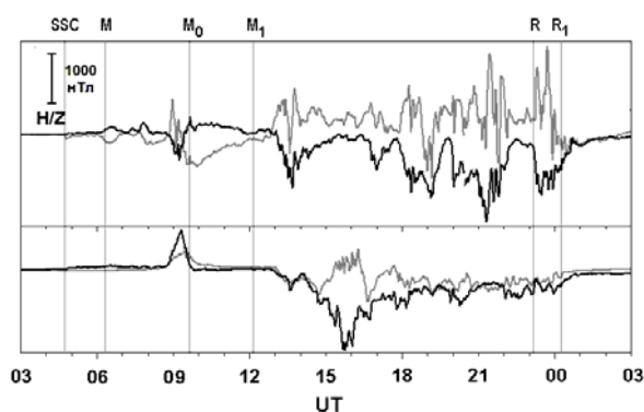
Рис. 11. Вариации H/Z -компонент геомагнитного поля в показанном на рис. 9 временном интервале, зафиксированные в \sim 30^\circ к востоку от поля зрения ЕКБ-радар магнитными обсерваториями TIK (вверху) и УАК (внизу)
