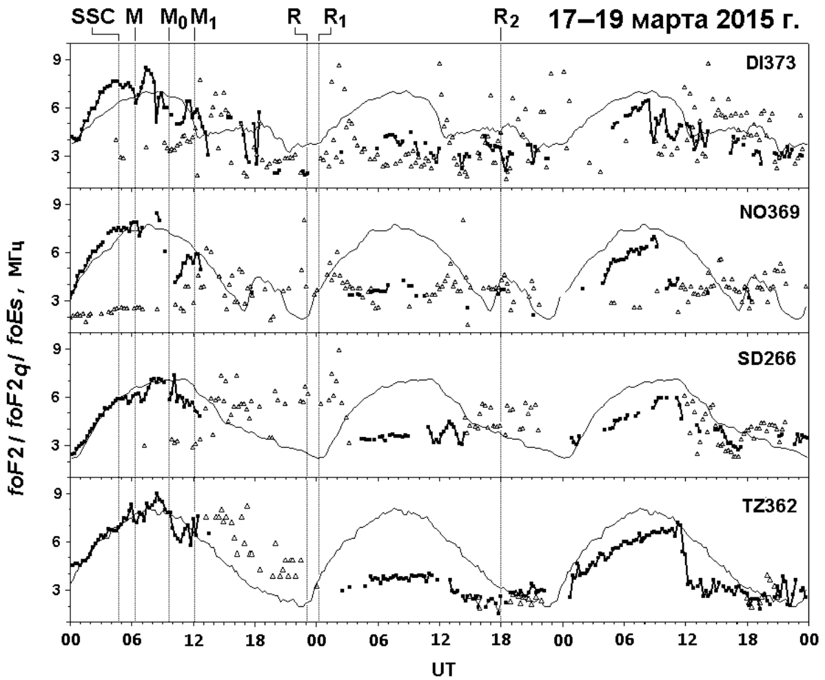
Рис. 5. Для 17–19 марта 2015 г. показаны вариации максимальной плазменной частоты слоев F2 ( f_oF2 ) и E ( f_oE_s ) ионосферы над тремя станциями, расположенными в секторе обзора ЕКБ-радара, и над ст. TZ362, находящейся в 6.3^\circ к югу от него. Вариации текущих значений f_oF2 показаны толстыми линиями и квадратами, фоновых — тонкими линиями, f_oE_s — треугольниками
