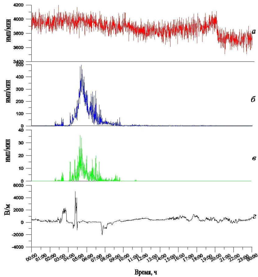
Рис. 3. Скорости счета нейтронов (а) и уровня электромагнитных помех, полученные при регистрации с различными порогами дискриминации усилителей 0.2 В (б) и 0 В (в) соответственно; напряженность электрического поля по данным флюксметра, установленного на станции КЛ «Иркутск-3000» (г) для 22 июня 2015 г.
