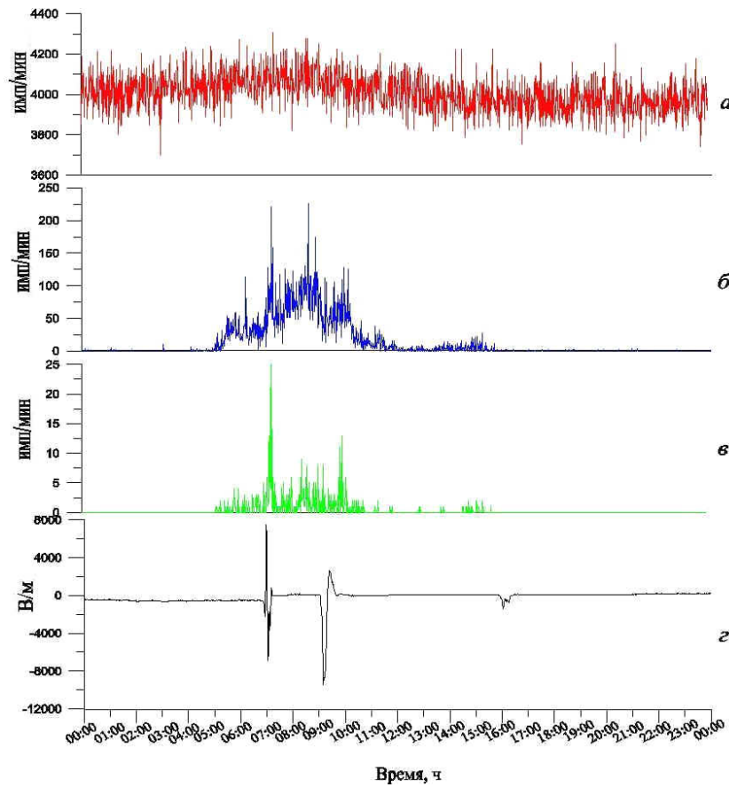
Рис. 1. Скорости счета нейтронов (а) и уровни электромагнитных помех, полученные при регистрации с различными порогами дискриминации усилителей 0.2 В (б) и 0 В (в) соответственно; напряженность электрического поля по данным флюксметра, установленного на станции КЛ «Иркутск-3000» (г) для 14 июня 2015 г.
