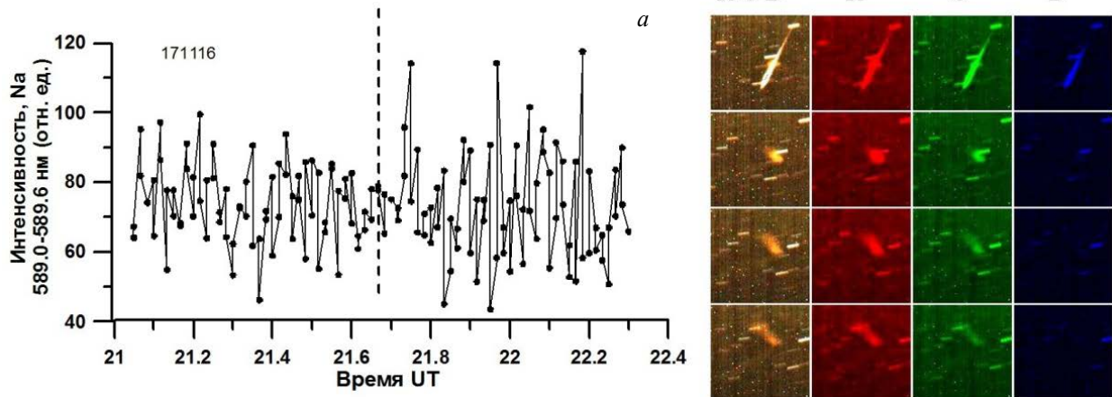
Рис. 2. Вариации интенсивности линий натрия Na 589.0-589.6 нм (а) и фрагменты кадров изображений из рис. 1, разделенных по цветовым каналам R-G-B (б). Вертикальной штриховой линией указано время взрыва метеороида
