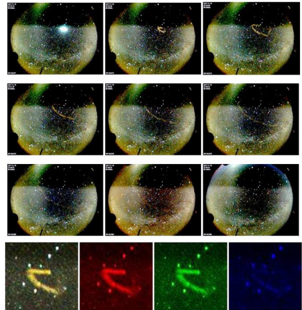
Рис. 4. Последовательные изображения, полученные 18 ноября 2017 г. цветной камерой в ССО в те же интервалы времени, что указаны на рис. 3. Нижний ряд: увеличенные фрагменты изображения в цветном и R-G-B-каналах для времени 22:25 UT
