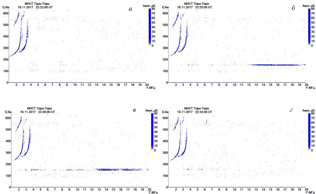
Рис. 5. Ионограммы вертикального зондирования, полученные Ионозондом-МС 18 ноября 2017 г.
