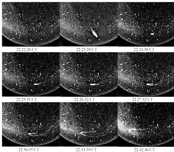
Рис. 3. Фрагменты изображений, полученных в ГФО 18 ноября 2017 г. камерой всего неба KEO Sentinel у западного горизонта
