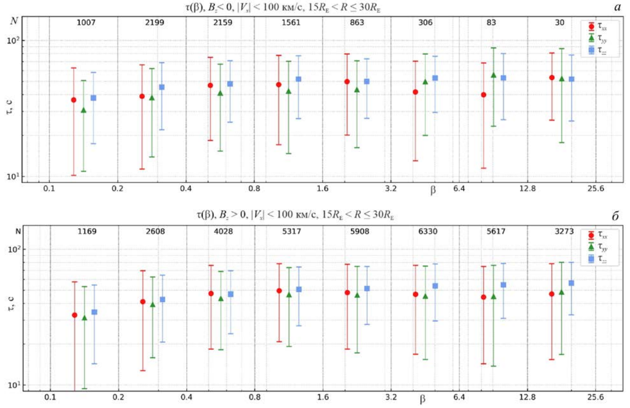
Рис. 5. Зависимость автокорреляционного времени \tau_{\text{auto}}(\beta) при B_z < 0 (a); B_z > 0 (б)
