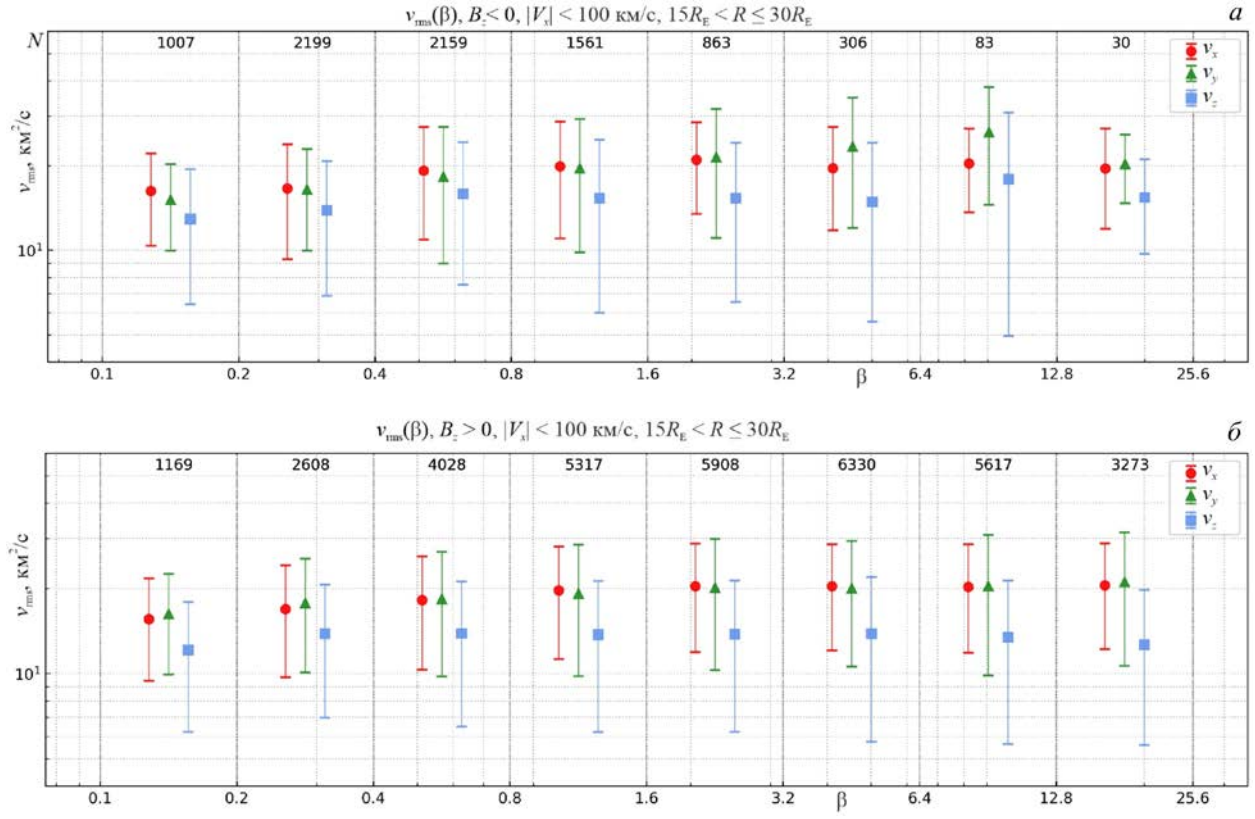
Рис. 3. Зависимость среднеквадратичной скорости v_{rms}(\beta) при B_z < 0 (a); B_z > 0 (б)
