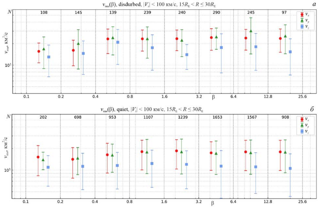
Рис. 4. То же, что на рис. 3, при SML < -200 \text{ нТл} (a); SML > -50 \text{ нТл} (б)
