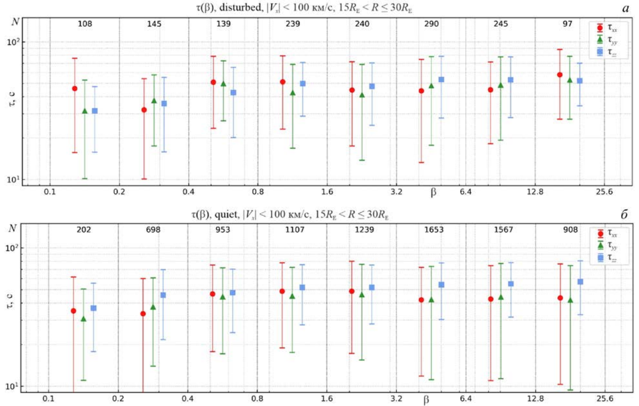
Рис. 6. То же, что на рис. 5, при SML < -200 нТл (a); SML > -50 нТл (б)
