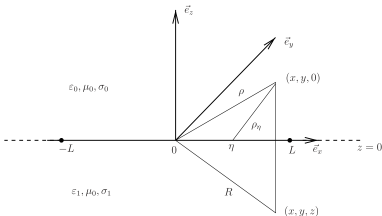
Рис. 1 — Геометрия задачи.
